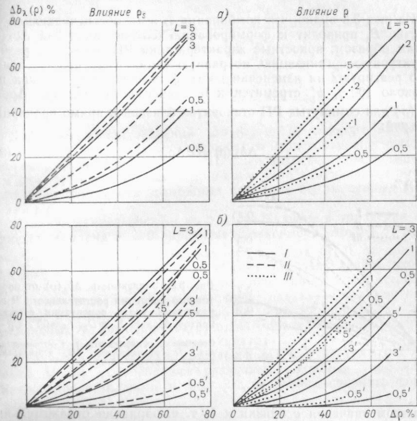
Рис. 3.2. Графики связи относительных изменений СКЯ РП, обусловленных изменением спектральных коэффициентов отражения отдельных фитоэлементов \Delta b_\lambda(\rho) , с относительными изменениями спектральных коэффициентов отражения отдельных фитоэлементов \Delta \rho . Надир, S_\lambda \gg D_\lambda , h_0 > 55^\circ , \tau/\rho = 0 .
