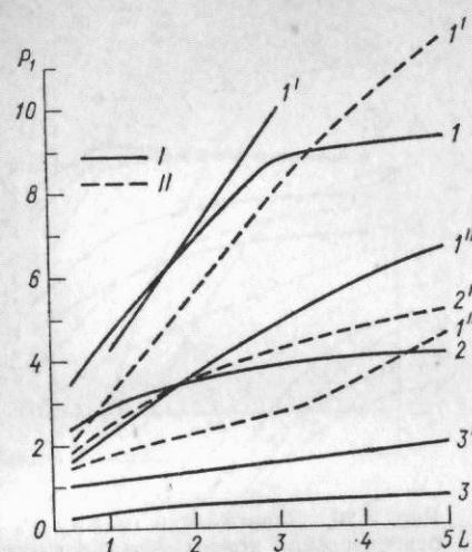
Рис. 3.23. Зависимость между P_i и относительной поверхностью фитоэлементов L . Надир, h_0=65^\circ , S_\lambda \gg D_\lambda .
