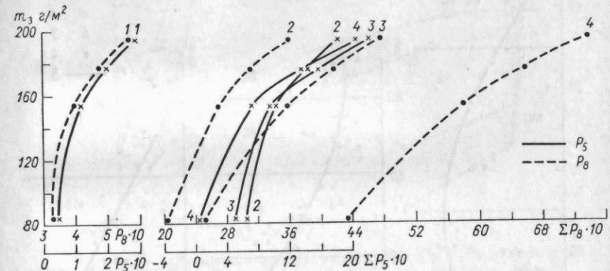
Рис. 5.10. Зависимость между P_5 , P_8 , их накопленными суммами \Sigma P_5 , \Sigma P_8 за различные периоды от фенофазы цветения до восковой спелости и запасами зерна m_3 в посевах яровой пшеницы. Степные районы Украины, h_0 > 45^\circ , ясная малооблачная погода, наземные измерения.
