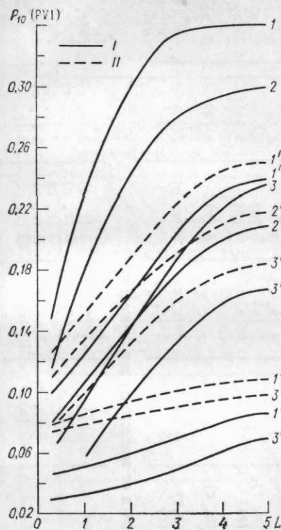
Рис. 3.29. Зависимость между P_{10} и относительной поверхностью фитоэлементов L . Надир, h_0=65^\circ , S_\lambda \gg D_\lambda .
