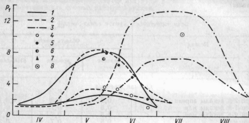
Рис. 5.5. Vegetационный ход расчетных (1—3, 8) и экспериментальных (4—7) значений P_1 для посевов различных культур плохого и хорошего состояний. Надир, полуденные часы.
