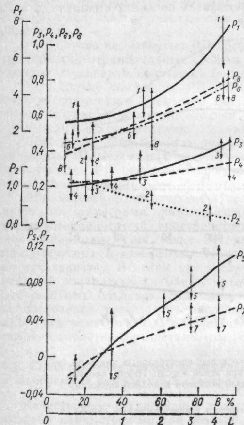
Рис. 4.3. Изменение комплексных спектральных индексов P_i в зависимости от проективного покрытия V и относительной поверхности фитоэлементов L посевов озимой пшеницы. Надир, полуденные часы, ясная малооблачная погода, фенофаза колошение—цветение, наземные измерения.
