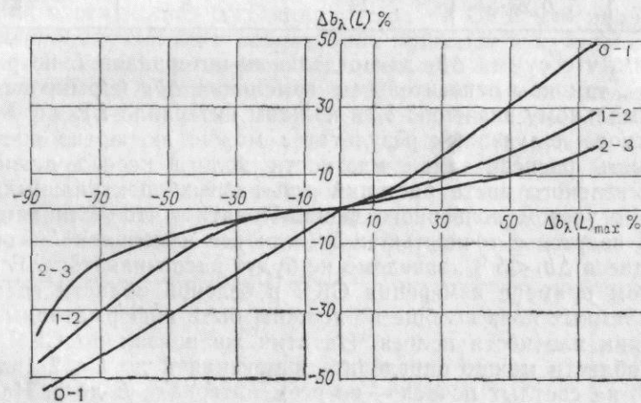
Рис. 5.3. Номограмма для определения \Delta b_\lambda(L) РП в различных интервалах L . Надир, S_\lambda \gg D_\lambda , h_\odot > 55^\circ , сферическая ориентация, \tau/\rho=1 .
