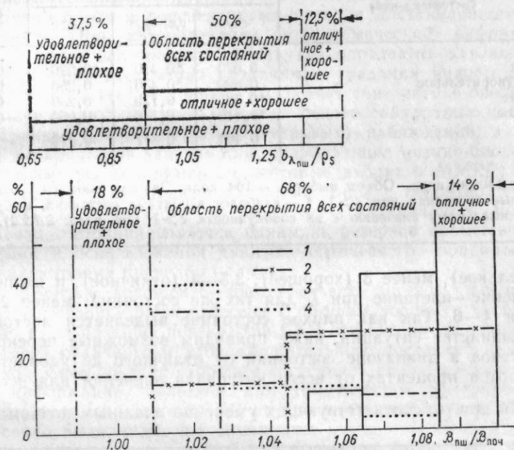
Рис. 5.9. Сопоставление рассчитанных по модели Гудриана b_{\lambda_{пш}}/\rho_s и измеренных по снимку «Ландсат» V_{пш}/V_{поч} относительных характеристик яркости в красной области видимого диапазона посевов озимой пшеницы в период молочно-восковой спелости. Степные районы Украины. Общий объем выборки около 100 полей: 1 — посеvy отличного состояния, 2 — хорошего, 3 — удовлетворительного, 4 — плохого.
