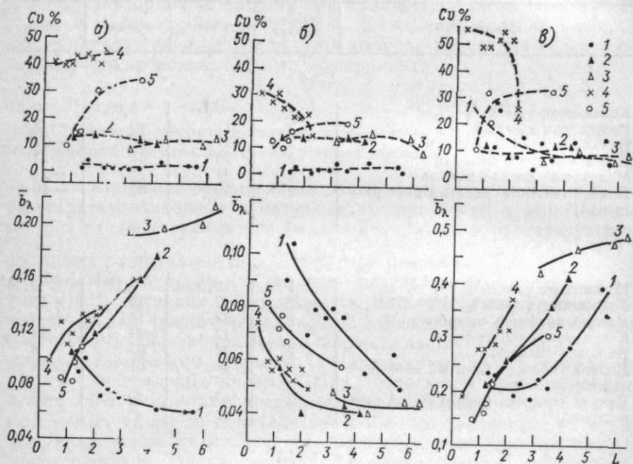
Рис. 4.1. Зависимость средних значений b_\lambda и их коэффициентов вариации Cv от L для посевов различных сельскохозяйственных культур. Надир, h_\odot > 45^\circ , наземные измерения.
