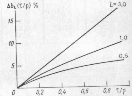
Рис. 3.4. Приращение значений b_\lambda РП за счет изменения прозрачности фитоэлементов ( \tau/\rho ) при сферической ориентации. Надир, S_\lambda \gg D_\lambda , h_\odot=65^\circ , \rho=0,15 .
