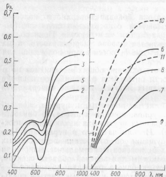
Рис. 2.3. Спектральные коэффициенты отражения \rho_\lambda листьев и стеблей озимой пшеницы Безостая I.
