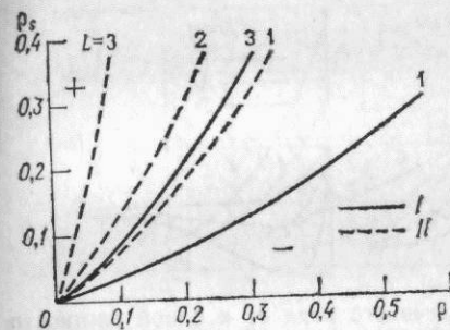
Рис. 3.13. График для определения типа дневного хода b_\lambda несомкнутых РП. Надир, S_\lambda \gg D_\lambda , сферическая ориентация фитозащитных элементов. I) \tau/\rho=0 , II) \tau/\rho=1 ; цифры у кривых—L; функция b_\lambda(h_\odot) возрастающая (+) и убывающая (—).
