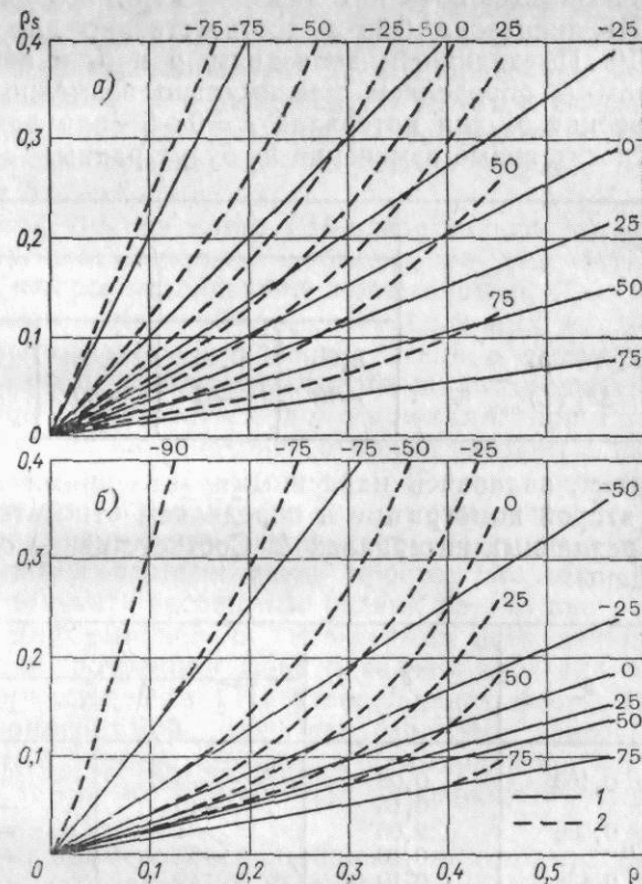
Рис. 5.2. Номограмма для определения максимально возможных изменений b_\lambda РП при увеличении L от 0 до 5 b_\lambda(L)_{\max} . Надир, S_\lambda \gg D_\lambda , h_\odot > 55^\circ .
