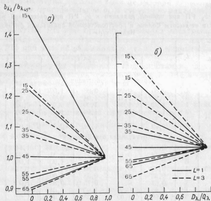
Рис. 3.19. Изменение функций приведения b_{\lambda} РП, измеренных при некоторой высоте Солнца ( b_{\lambda_i} ), к b_{\lambda} при h_{\odot}=45^{\circ} ( b_{\lambda_{45^{\circ}}} ) в зависимости от соотношения прямой и рассеянной радиации в облучающем потоке. Надир, сферическая ориентация фитоэлементов, \tau/\rho=1 .
