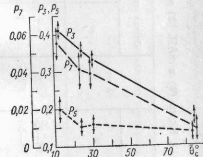
Рис. 4.5. Зависимость P_3 , P_5 , P_7 от среднего угла наклона стеблей \theta_c в посевах пшеницы (описание объекта см. в табл. 4.3А). Надир, полуденные часы, ясная малооблачная погода, наземные измерения.
