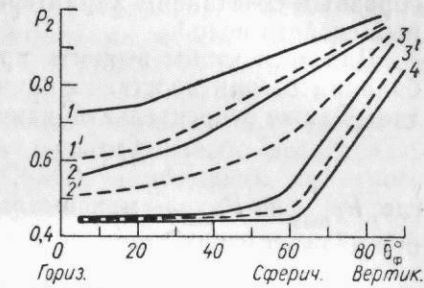
Рис. 3.21. Зависимость между P_2 и средним углом наклона фитоэлементов \theta_\phi для зеленой растительности. Надир, h_\odot=65^\circ , S_\lambda \gg D_\lambda , \rho_k=0,075 , \rho_a=0,15 ; \rho_{sk}=0,15 , \rho_{s3}=0,15 (светлые почвы); \rho_{sk}=0,06 , \rho_{s3}=0,06 (темные почвы).
