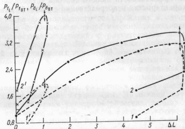
Рис. 5.12. Зависимость между отношением P_1 и P_8 в фиксированные сроки ( P_{1i} и P_{8i} ) к P_1 и P_8 для фенофазы выход в трубку ( P_{1VT} и P_{8VT} ) и приращением относительной поверхности фитоэлементов \Delta L за период от выхода в трубку до фиксированного срока для посевов озимой пшеницы разного состояния.
