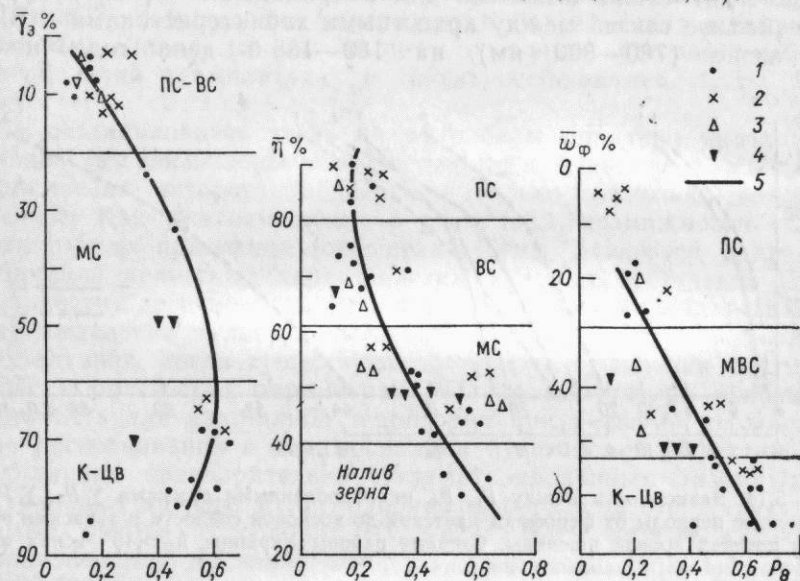
Рис. 5.11. Зависимость между P_8 и долей относительной поверхности фитоэлементов зеленого цвета \gamma_z , содержанием сухого вещества в зерне \eta и обводненностью фитоэлементов \phi_w для посевов озимой пшеницы в период фенофаз от колошения до полной спелости. Надир, полуденные часы, ясная малооблачная погода, наземные измерения.
