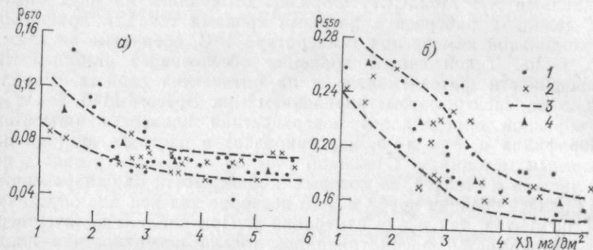
Рис. 2.2. Изменение \rho_\lambda листьев райграса итальянского в зависимости от поверхностной плотности хлорофилла.
