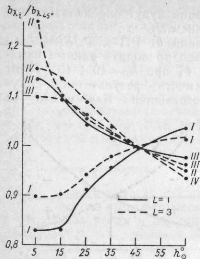
Рис. 3.18. Функции приведения b_{\lambda} , измеренных при некоторой высоте Солнца ( b_{\lambda_i} ), к b_{\lambda} при h_{\odot}=45^{\circ} ( b_{\lambda_{45^{\circ}}} ). Надир, S_{\lambda}=0,6 , D_{\lambda}=0,4 , сферическая ориентация фитоэлементов, \tau/\rho=1 .
