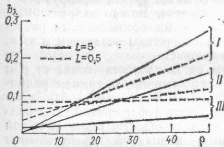
Рис. 3.1. Зависимость b_\lambda РП от спектральных коэффициентов отражения отдельных фитоэлементов \rho . Надир, S_\lambda \gg D_\lambda , h_0 = 65^\circ , \tau/\rho = 0 .
