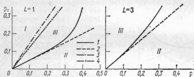
Рис. 3.10. График для определения типа связи b_\lambda РП со средним углом наклона фитоэлементов \bar{\theta}_\phi . Надир, S_\lambda \gg D_\lambda , h_0 = 65^\circ .
