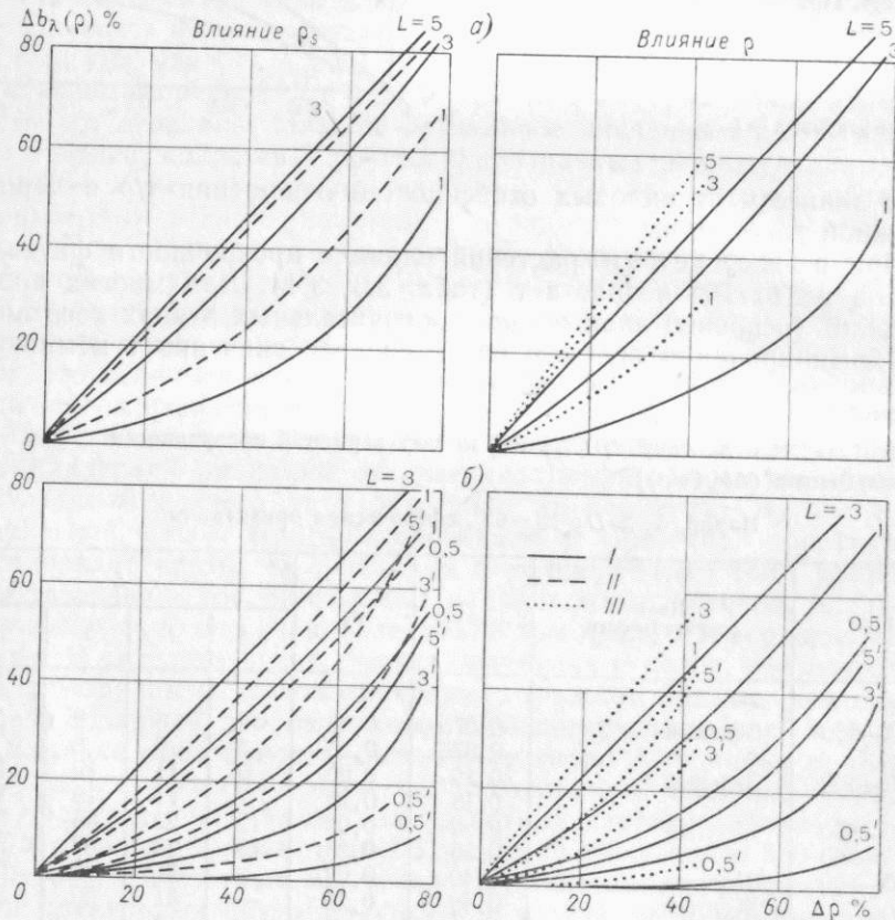
Рис. 3.5. Графики связи \Delta b_\lambda(\rho) с \Delta \rho . Надир, S_\lambda \gg D_\lambda , h_\odot > 55^\circ , \tau/\rho = 1 .
