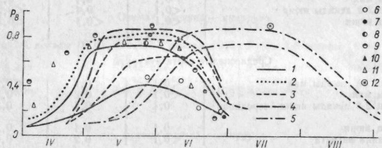
Рис. 5.6. Vegetационный ход расчетных (1, 3, 5, 12) и экспериментальных (2, 4, 6—11) значений P_8 для посевов различных культур плохого и хорошего состояний. Надир, полуденные часы.
