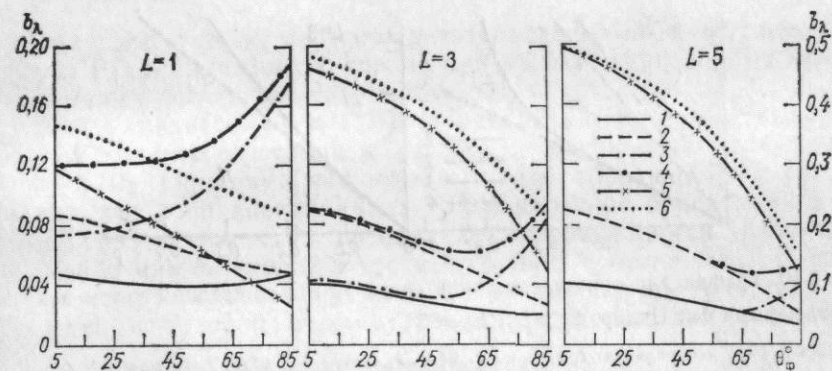
Рис. 3.9. Зависимость b_\lambda РП от среднего угла наклона фитоэлементов \bar{\theta}_\Phi . Надиr, S_\lambda \gg D_\lambda , h_0 = 65^\circ , \tau/\rho = 1 .
