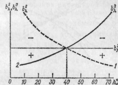
Рис. 3.17. Соотношение СКЯ при прямой ( b_\lambda^S ) и рассеянной ( b_\lambda^D ) радиации.
