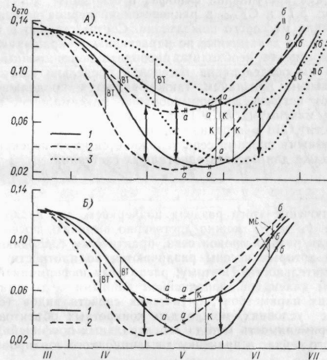
Рис. 5.7. Вегетационный ход расчетных значений СКЯ в красной области видимого диапазона ( b_{670} ) посевов озимой пшеницы в различных пунктах Украины. Надир, D_{\lambda}/Q_{\lambda}=0,4 , полуденные часы.
