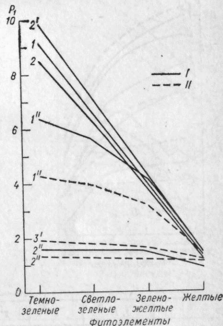
Рис. 3.25. Изменение P_i в зависимости от цвета растительности при разной плотности полога. Надир, h_0=65^\circ , S_\lambda \gg D_\lambda .
