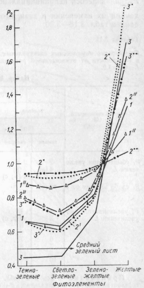
Рис. 3.22. Изменение P_2 в зависимости от цвета растительности при разной плотности полога РП. Надир, h_\odot=65^\circ , S_\lambda \gg D_\lambda .
