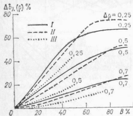
Рис. 3.3. Зависимость \Delta b_\lambda(\rho) от проективного покрытия растительности B при различных типах ориентации фитоэлементов. Надир, S_\lambda \gg D_\lambda , h_\odot = 65^\circ , \tau/\rho = 0 .
