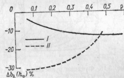
Рис. 3.14. Зависимость амплитуды дневного хода \Delta b_\lambda(h_\odot) сомкнутых РП от \rho . Надир, S_\lambda \gg D_\lambda , сферическая ориентация фитозащитных элементов. I) \tau/\rho=0 , II) \tau/\rho=1 .
