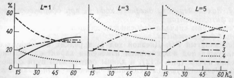
Рис. 3.12. Зависимость доли видимых освещенных и затененных участков почвы и растительности (%) от высоты Солнца h_\odot . Надир, сферическая ориентация фитоэлементов.
