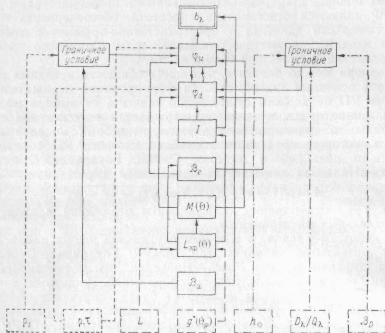
Рис. 1.1. Блок-схема модели отражения системы растительность—почва Гюдрриана.
