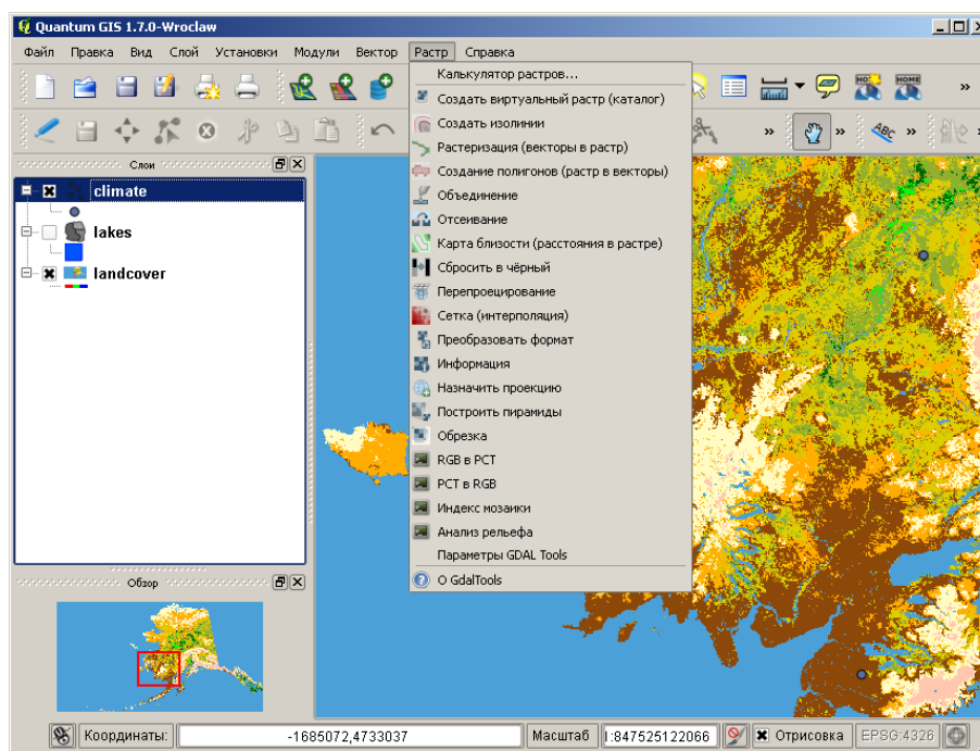
Рис. 12.13.: Меню Растр
