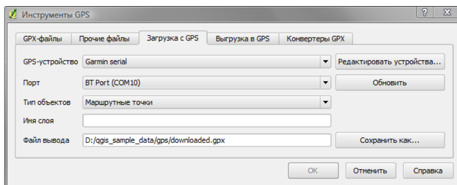
Рис. 12.22.: Инструмент загрузки
