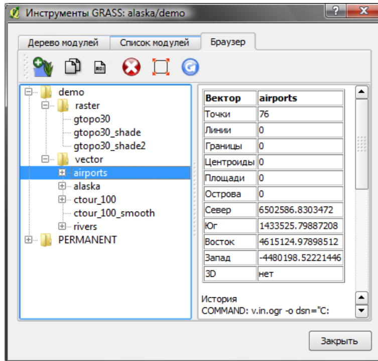
Рис. 9.14.: Браузер GRASS
