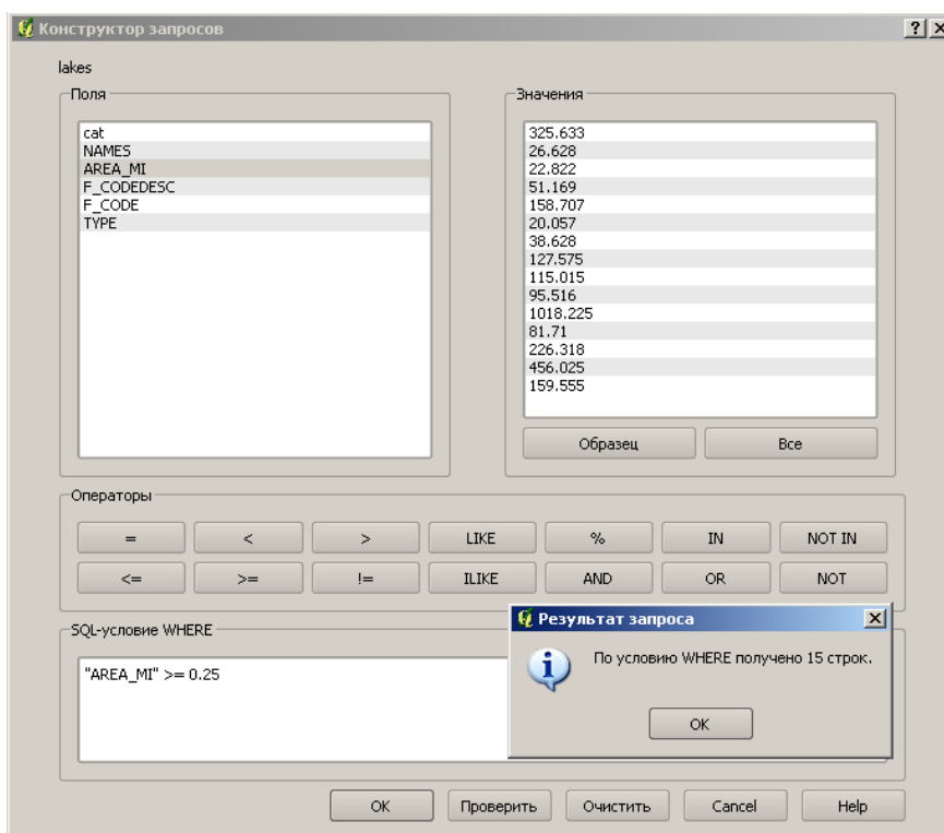
Рис. 4.32.: Конструктор запросов
